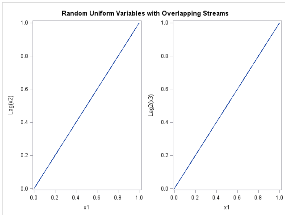
図 1.5 CALL RANUNI で異なるシードを使用する: 重複するストリームを持つランダムな一様分布変数:プロット 2
