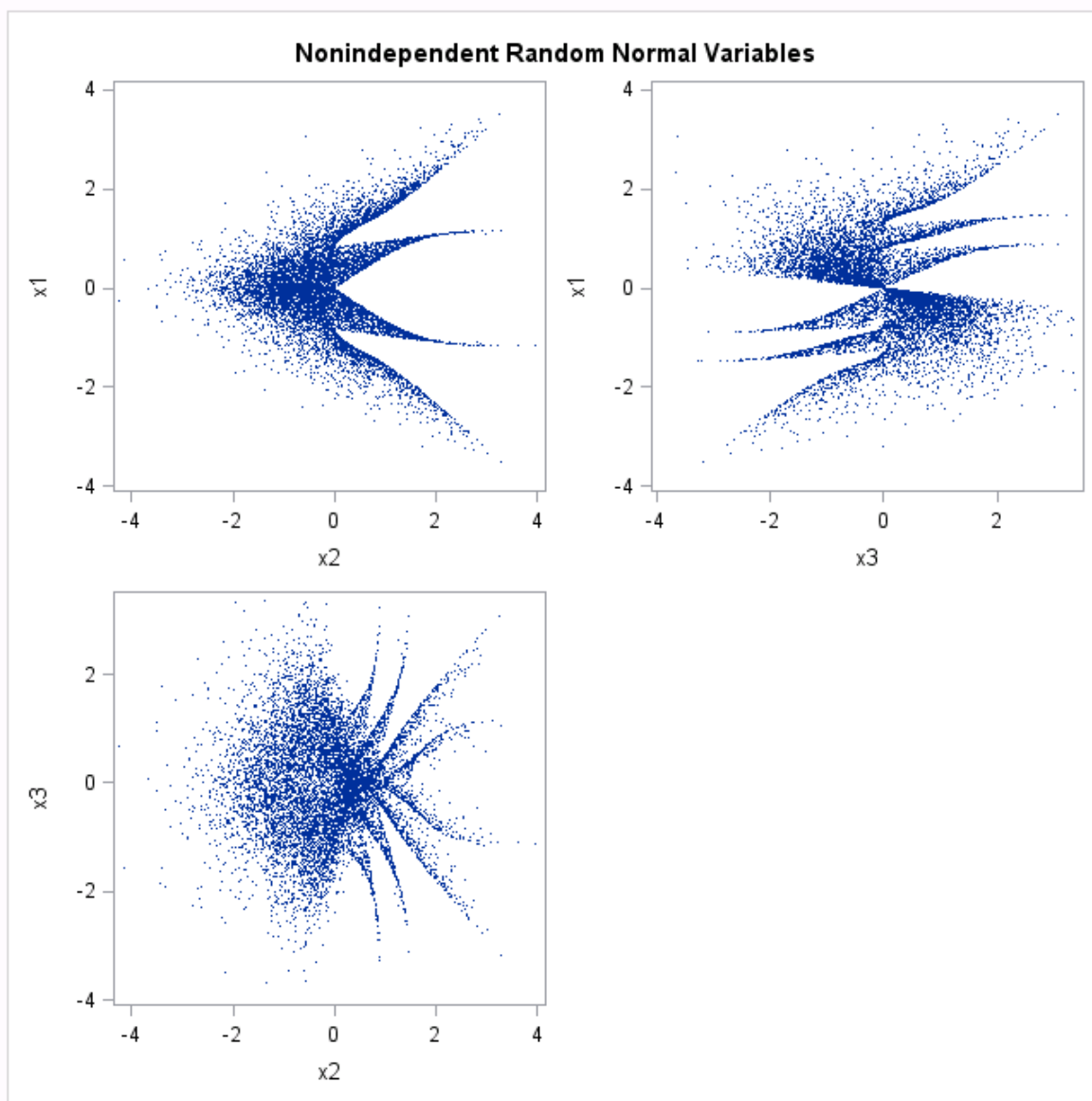
図 1.2 複数のシードから作成した複数のストリームの: 独立していないランダムな正規変数
