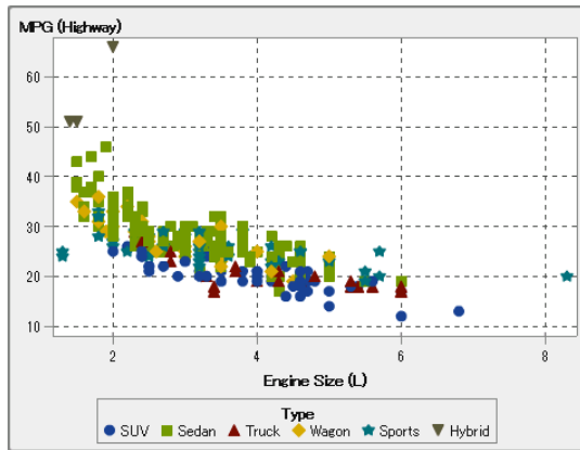
画面 A1.8 散布図
