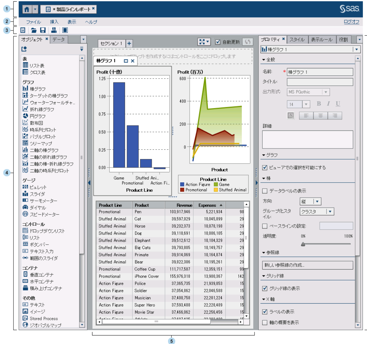
図 31.1 デザイナ
