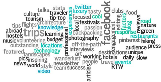
Новые предикторы
